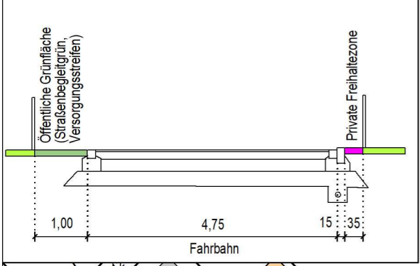
Schnitt A - B M 1 : 100
